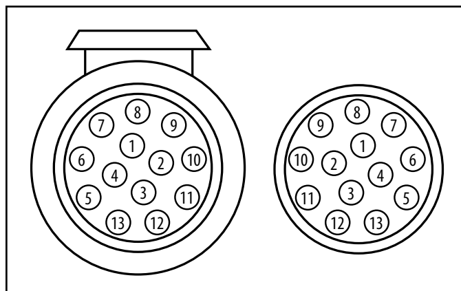
Figure 2 : Raccordement électrique à 13 broches
