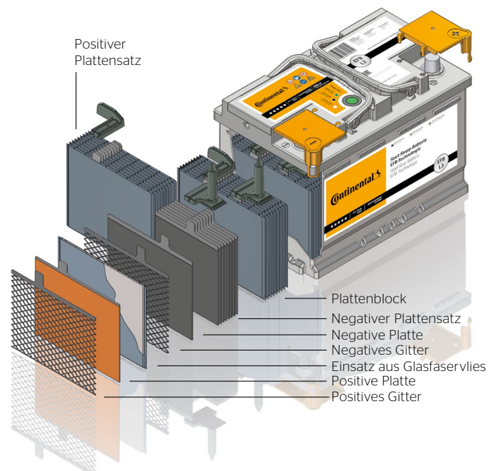
EFB-Technologie: Batterieaufbau
